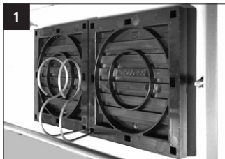
1 Innenansicht mit Lautsprecheradapter und Befestigungsbügel
