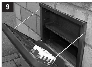
Haltestäbe einhängen, Elektroanschlüsse vornehmen, falls gegeben.
