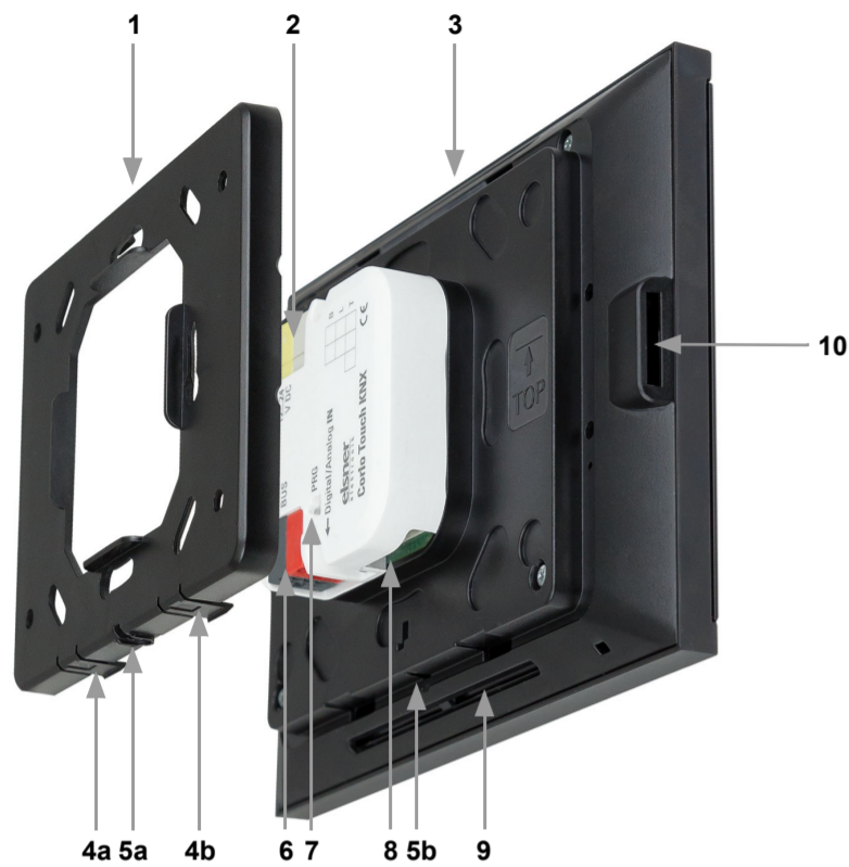
Abb. 8 1 Montage-Einheit 2 Klemme Hilfsspannung 24 V DC ±10%, Klemmenbelegung polungsunabhängig (+/- oder -/+) 3 Displayeinheit 4 Rasten für Schnappverschluss 5 Öffnung für Schraube (Fixierung) 6 KNX-Klemme Bus +/- 7 Programmier-Taster zur Adressierung des Geräts am Bus (versenkt) 8 Buchse Analog/Digital-Eingänge 9 Belüftungsschlitze 10 Micro SD-Buchse (Kontakte der Karte müssen beim Einlegen Richtung Display weisen)
