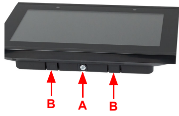
Abb. 7 Zum Abnehmen der Displayeinheit von der Montage-Einheit lösen Sie die Schraube (A). Drücken Sie gegen die unteren Rasten (B), um die Verbindung zu lösen. Die Displayeinheit kann entnommen werden.
