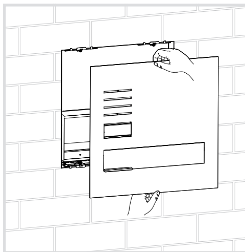
Bild 13: Briefkastenfront einsetzen
