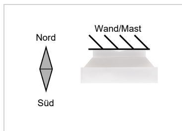
Abb. 3 Bei Installation auf der Nordhalbkugel muss das Gerät nach Süden ausgerichtet werden.
