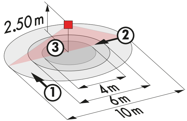
Reichweitendiagramm
