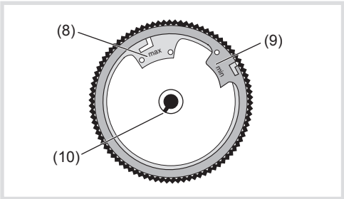
Bild 5: Regulierknopf von hinten
