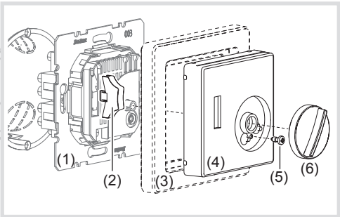
Bild 1: Geräteaufbau
