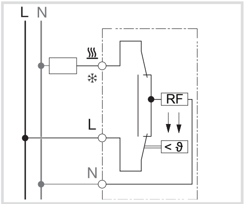
Figura 4: Collegamenti elettrici
