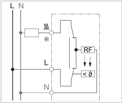
Bild 4: Elektrischer Anschluss
