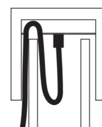
Abb. 10b: Querschnitt des Sockels. Leitung zwischen Sockel und Mast nach Außen führen
