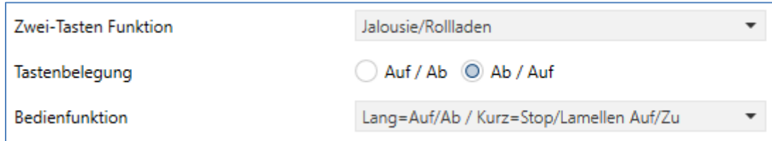
Abbildung 79: Jalousie
