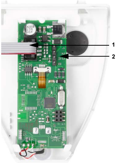
Abb. 12: Übersicht Platine
