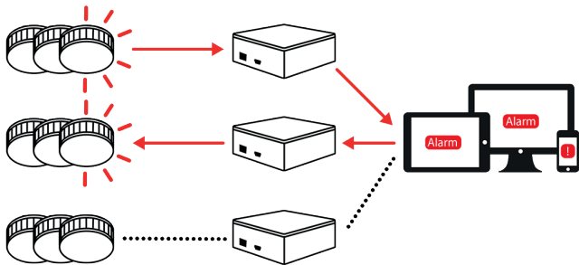
Abb. 4 Gateway-zu-Gateway-Schaltung/Alarmweiterleitung
