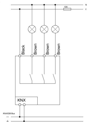
Anschlussbeispiel AKK-03UP.03
