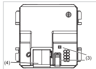
Bild 2: Rückansicht Taster-Modul
