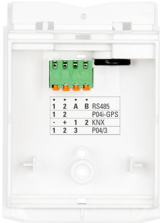
Abb. 14 Schließen Sie Steuerung/Spannung (+24 V DC/GND) an den Klemmen 1/2 P04i-GPS an.
