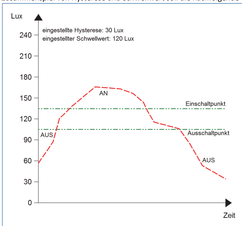
Abbildung 5: Hysterese Schwellwertschalter
