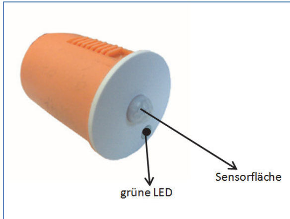
Abbildung 2: Hardwaremodul
