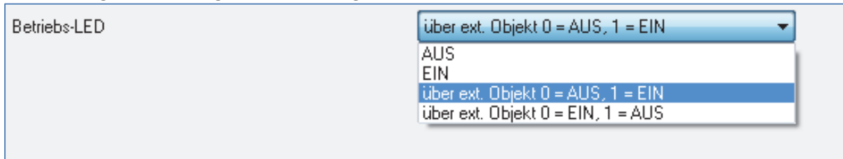
Abbildung 25: Konfiguration Betriebs LED
