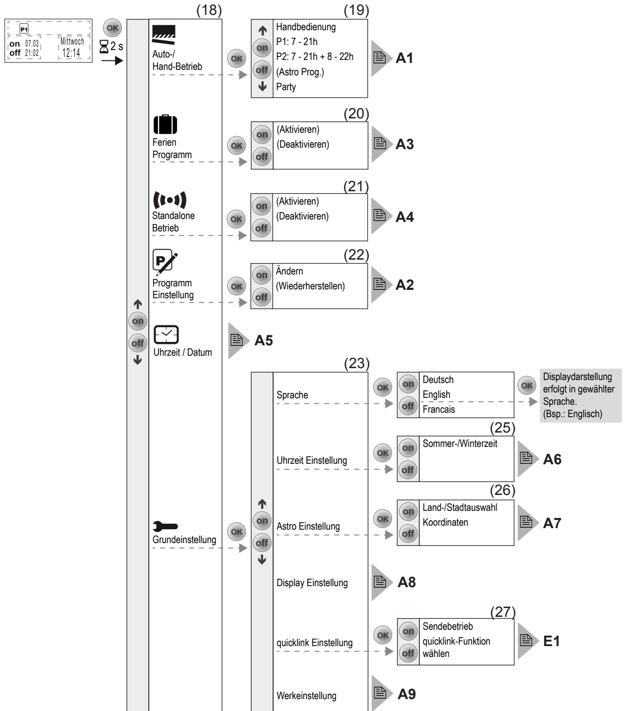
Bild 4: Menü-Übersicht
