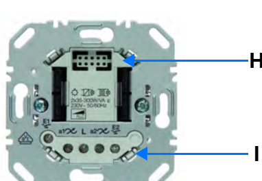
2 Ausgänge Dimmer
