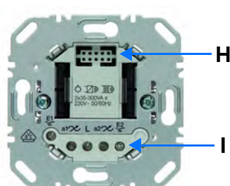
2 Ausgänge Umschaltung
