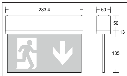
S1 (Maße in mm)
