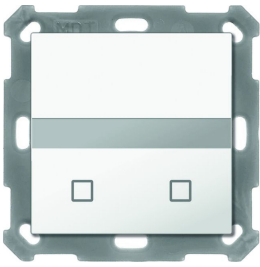
MDT KNX 55 x 55 mm Bewegungsmelder mit Temp.sensor reinweiß matt Up
