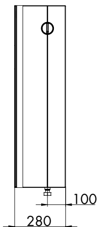
Seitenansicht rechts
