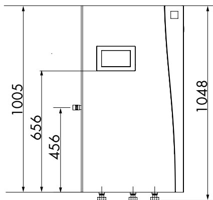
Frontansicht
