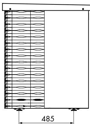
Seitenansicht links
