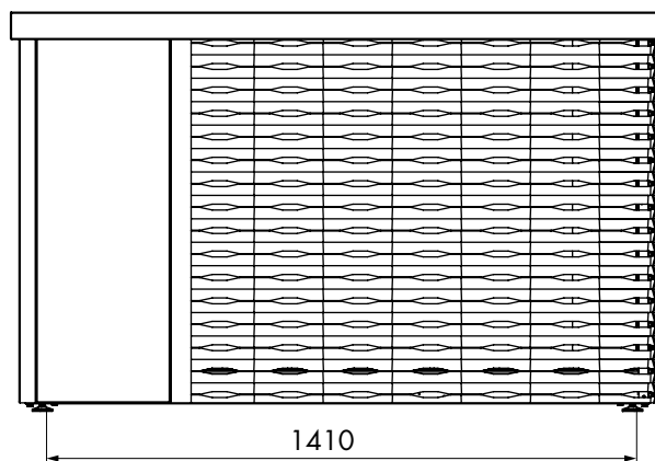
Rückansicht (Ansaugseite)
