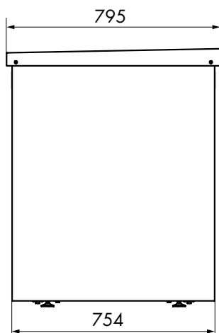
Seitenansicht rechts
