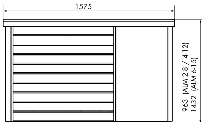
Frontansicht (Ausblasseite)
