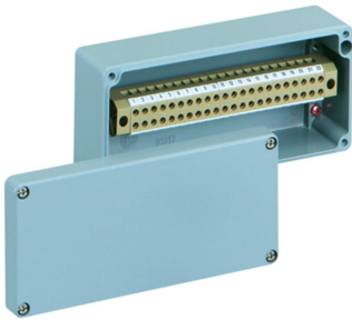
SPELSBERG Alu-Reihenklemm-Gehäuse ALR 1808-4 mit Klemmen
