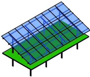
SL Rack Freilandaufständerung 3V-20 Grad-9
