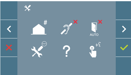
Bildschirm: ADMINISTRATORMENÜ
