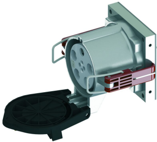
R&amp;S Anbausteckdose FCP FCP-S4/250 400V-6h
