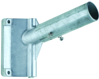
Alu-Mehrzweck-Rohrausleger, lackiert Dm 60x250mm
