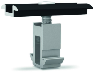
K2 DomeClamp Mittelklemme 30-50 mm schwarz eloxiert
