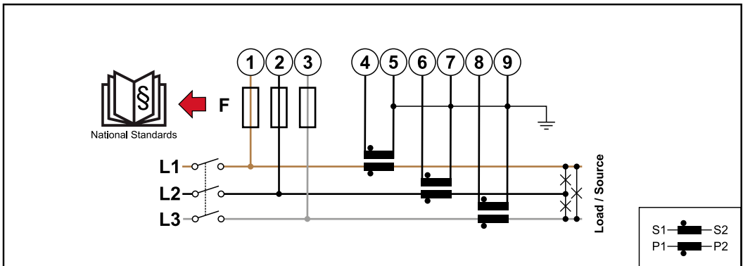
3 Phasen, 3 Leiter (CT-Anschluss)
