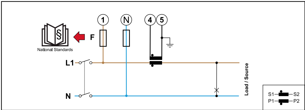
1 Phase, 2 Leiter (CT-Anschluss)
