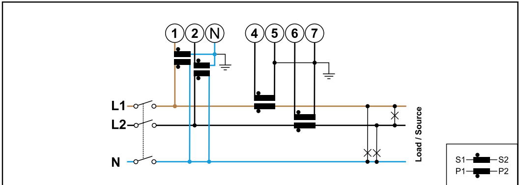
2 Phasen, 3 Leiter (VT/CT-Anschluss)
