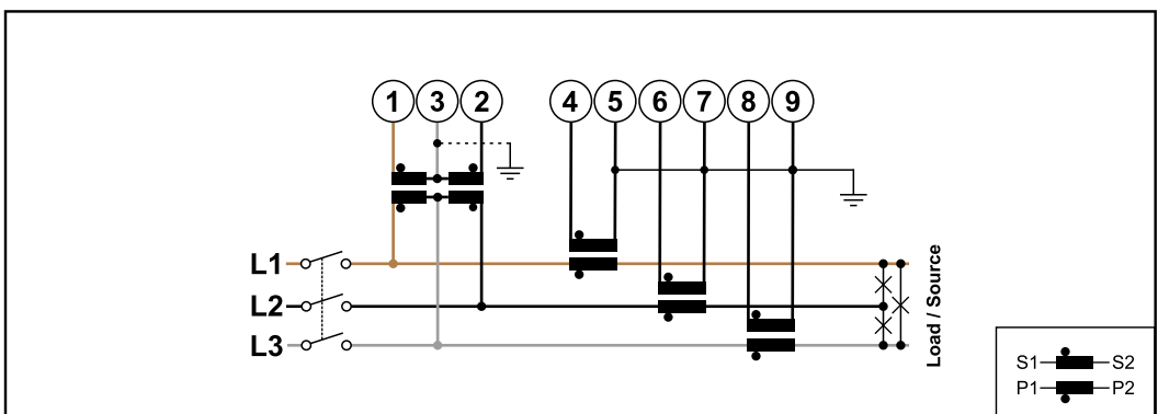
3 Phasen, 3 Leiter (VT/CT-Anschluss)
