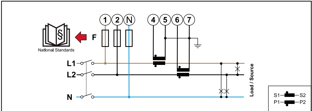
2 Phasen, 3 Leiter (CT-Anschluss)
