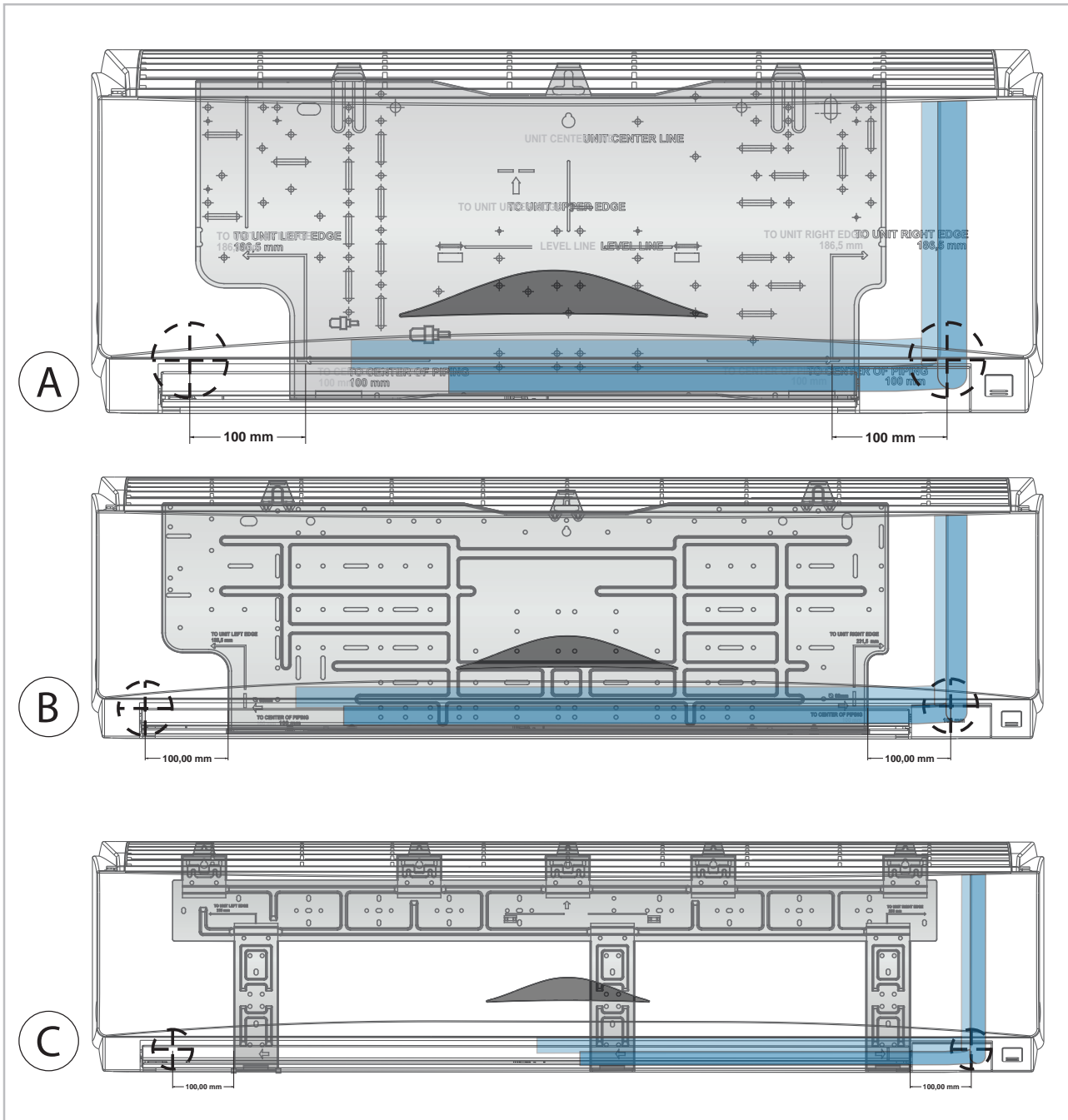
Abb. 29: Montageplatten
