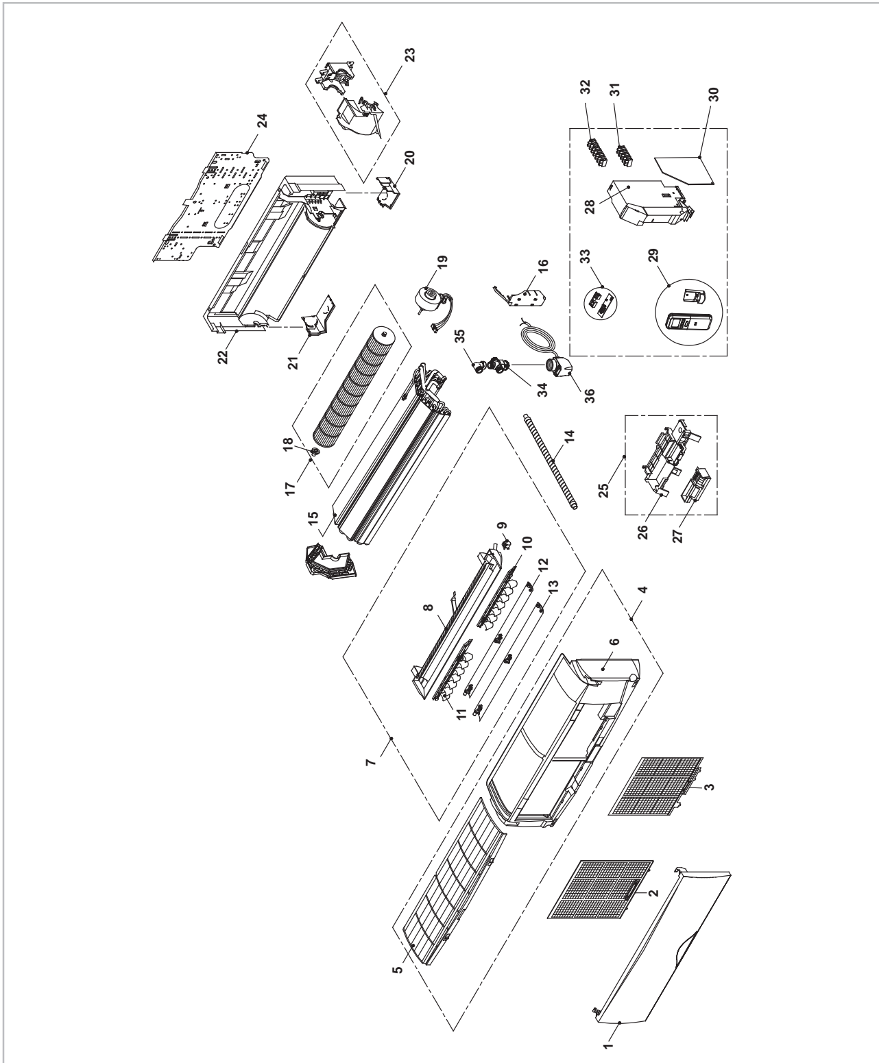
Abb. 40: Gerätedarstellung
