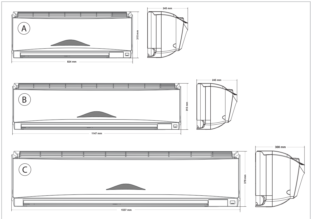
Abb. 1: Geräteabmessungen
