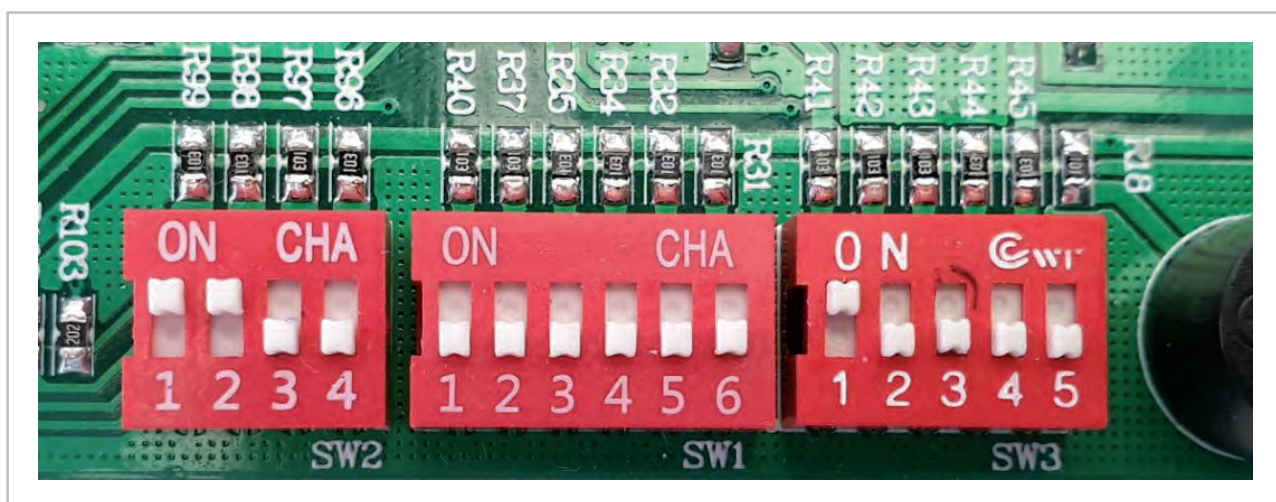
Abb. 35: DIP-Schalterblöcke SW1-SW3
