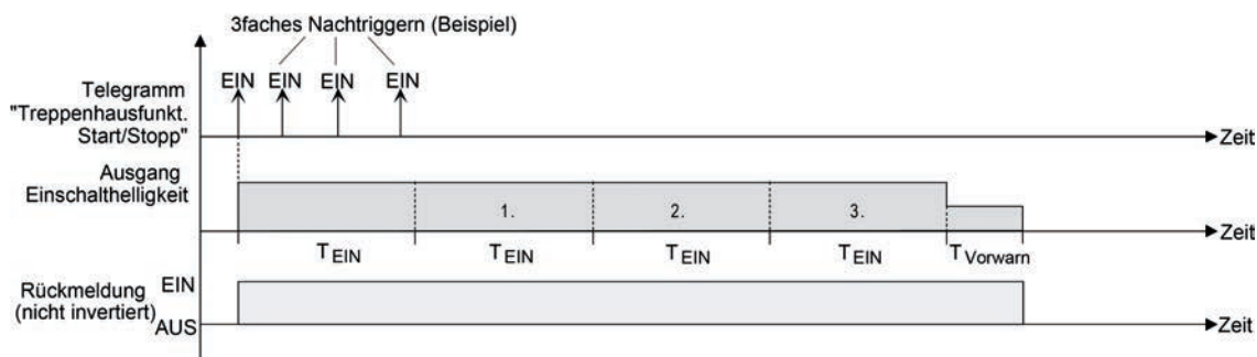
Bild 51: Zeitverlängerung der Treppenhausfunktion
