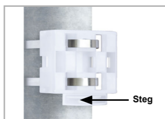
Abb. 5 Bei Mastmontage: geschwungene Seite zum Mast, Steg nach unten.
