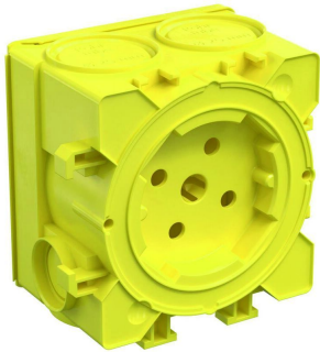
B2 Geräte Verbindungsdose System Haftmag Einbau. Ø 60 mm, Tiefe 48,5 mm
