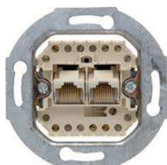
UAE Steckdose 8/8-polig, Cat.3
